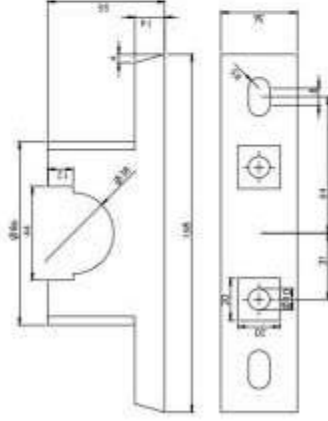
1) Base body
